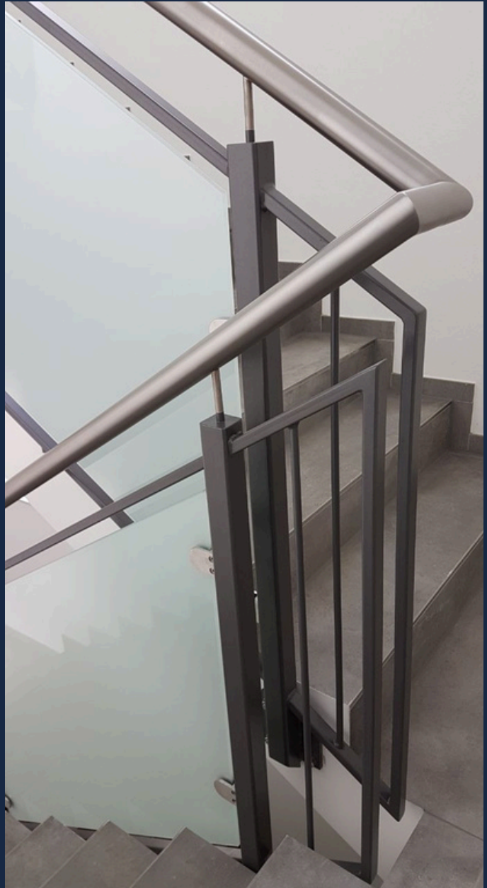
Geländer-Konstruktion in Stahl pulverbeschichtet - Handlauf in Edelstahl - Geländerfüllung aus VSG matt sowie senkrechtem Stab -Kombination aus Rund-und Vierrkantprofilen
